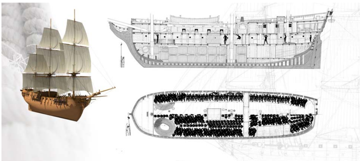
Plans du navire négrier « L'Aurore ». Source : Guy Ribadeau-Dumas Architecte naval.
